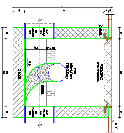
DETALJ REVIZIJSKOG ODOBRSKOG I PEŠAKNOG OKNA PRESJEK 1-1 M 1:20
