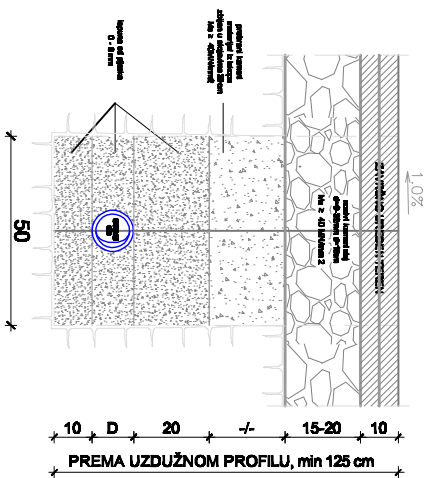
POPRERNI PRESJEK NOVA VODOSTAVNOG ODVOJILNICA D 110x90 mm M 1:20
