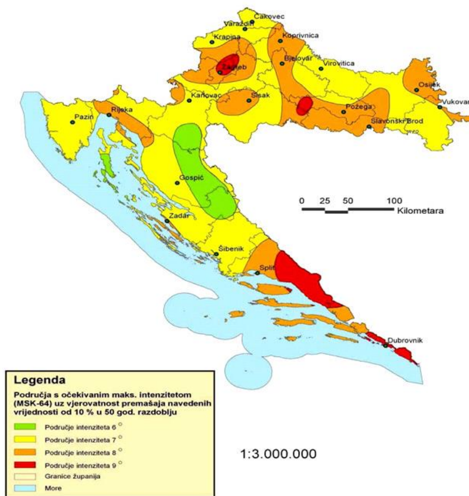
Slika 5. Seizmološka karta Hrvatske;
