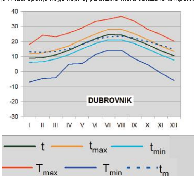
Slika 9. Godišnji hod srednje ( t ), srednje minimalne ( t_{\min} ) i maksimalne ( t_{\max} ) i apsolutne minimalne ( T_{\min} ) i maksimalne ( T_{\max} ) temperature zraka i temperature mora ( t_m ), °C Izvor: Klimatski atlas Hrvatske 1961.-1990., 1971. -2000.
