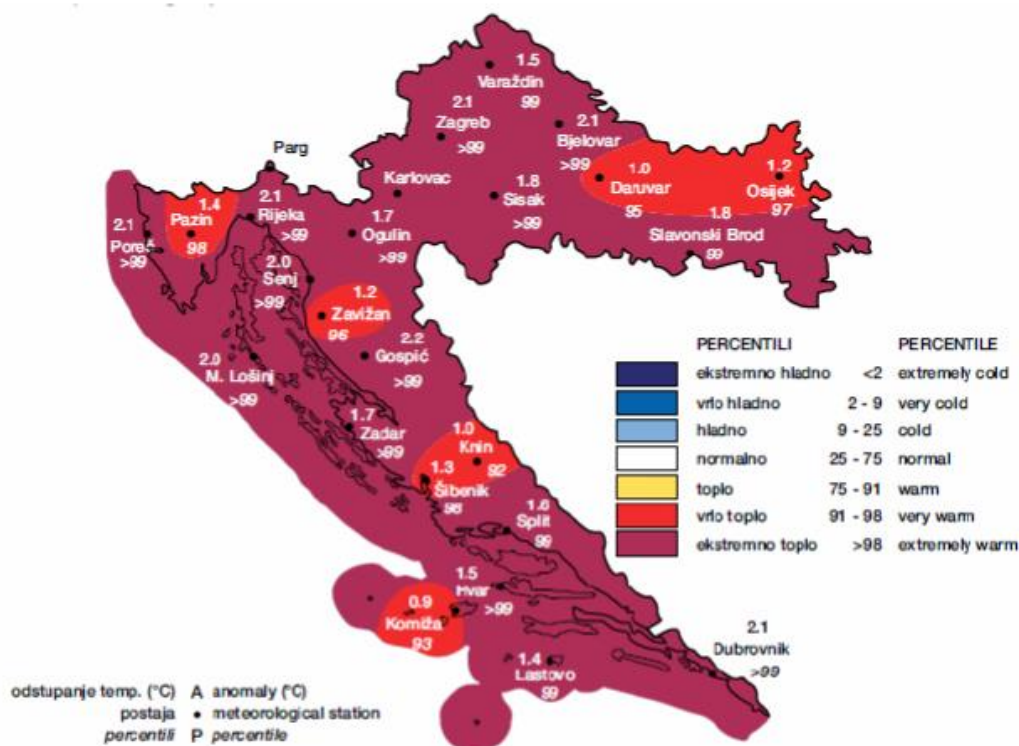
Slika 11. Odstupanje srednje sezonske temperature zraka ( ^{\circ}\text{C} ) od višegodišnjeg prosjeka za razdoblje 1961. – 1990. Godina za Hrvatsku za ljetu 2016. Godine (lipanj – kolovoz), Izvor: Praćenje i ocjena klime u 2016. godini
