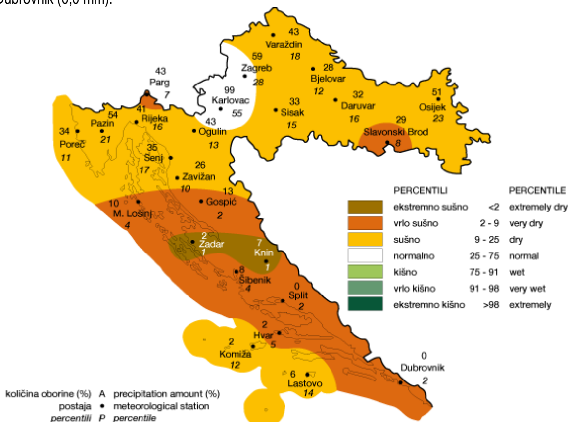
Slika 13. Odstupanje količine oborine za kolovoz 2017. izrađene u postocima višegodišnjeg prosjeka (1961.-1990.)
