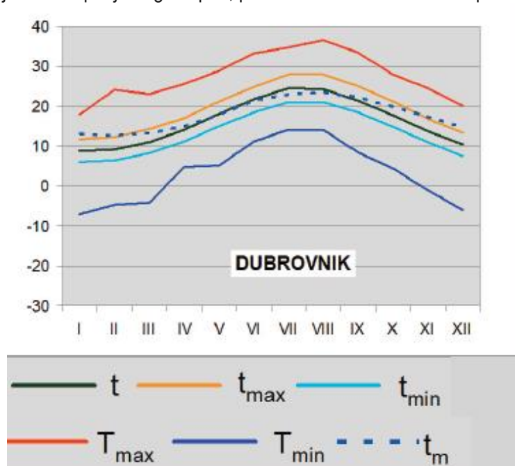
Slika 9. Godišnji hod srednje ( t ), srednje minimalne ( t_{min} ) i maksimalne ( t_{max} ) i apsolutne minimalne ( T_{min} ) i maksimalne ( T_{max} ) temperature zraka i temperature mora ( t_m ), °C Izvor: Klimatski atlas Hrvatske 1961.-1990., 1971.-2000.
